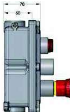
Vista lateral
