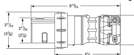
60A Plug
