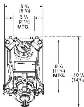
30A Plug
