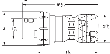
30A Plug
