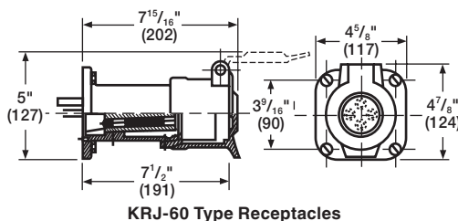
KRJ-60 Type Receptacles
