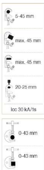
MPL Pinza de media tensión
